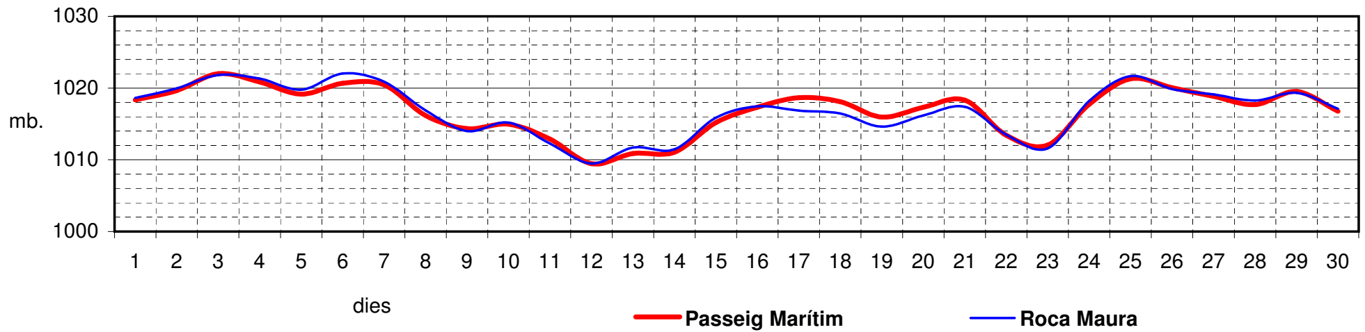
L'Estartit - Pressió atmosfèrica reduïda al nivell del mar - juny 2015
