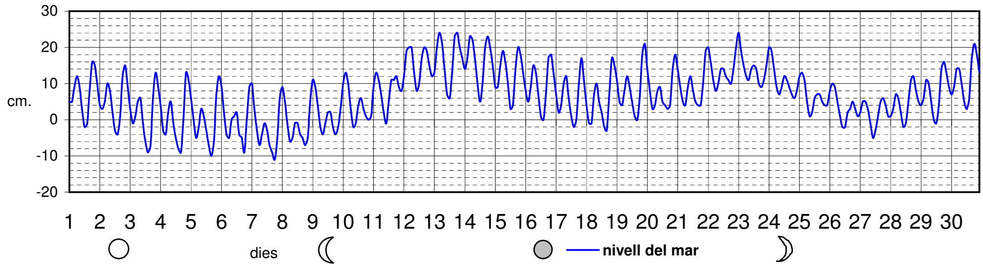
L'Estartit - marea - juny 2015
