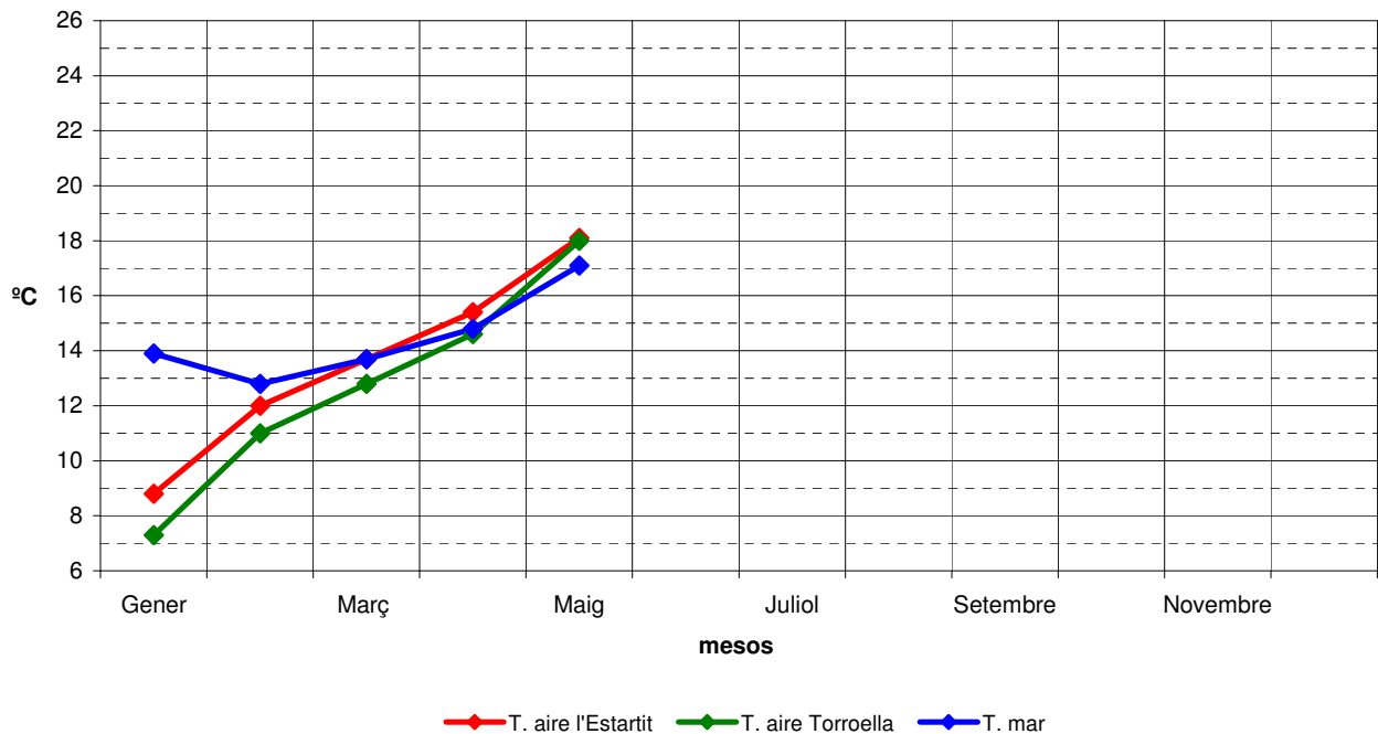
Temperatures mitjanes de l'aire a l'Estartit i Torroella i del mar en superfície, any 2017
