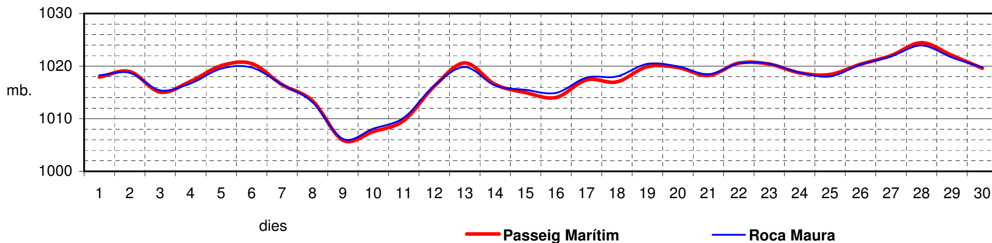
L'Estartit - Pressió atmosfèrica reduïda al nivell del mar - setembre 2017
