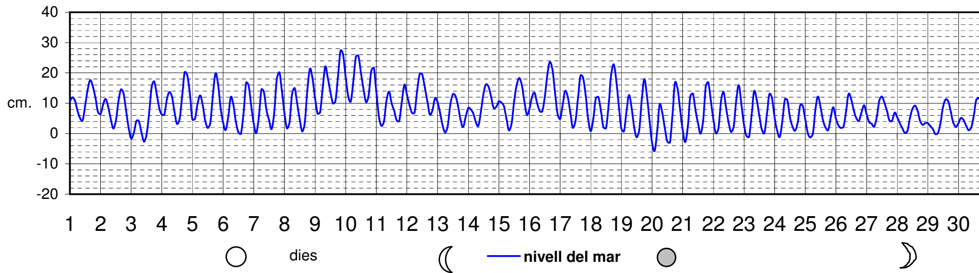
L'Estartit - marea - setembre 2017
