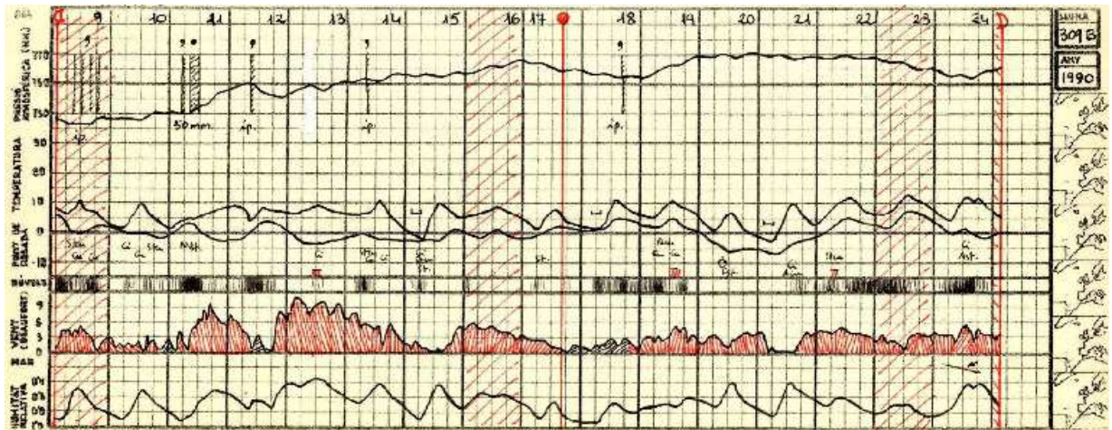
Meteograma d'aquells dies a l'Estartit. Es pot observar, a l'apartat del vent, un domini dels colors vermells que indiquen vents de component nord. També, com el màxim de vent va ser durant la matinada del dia 13.
