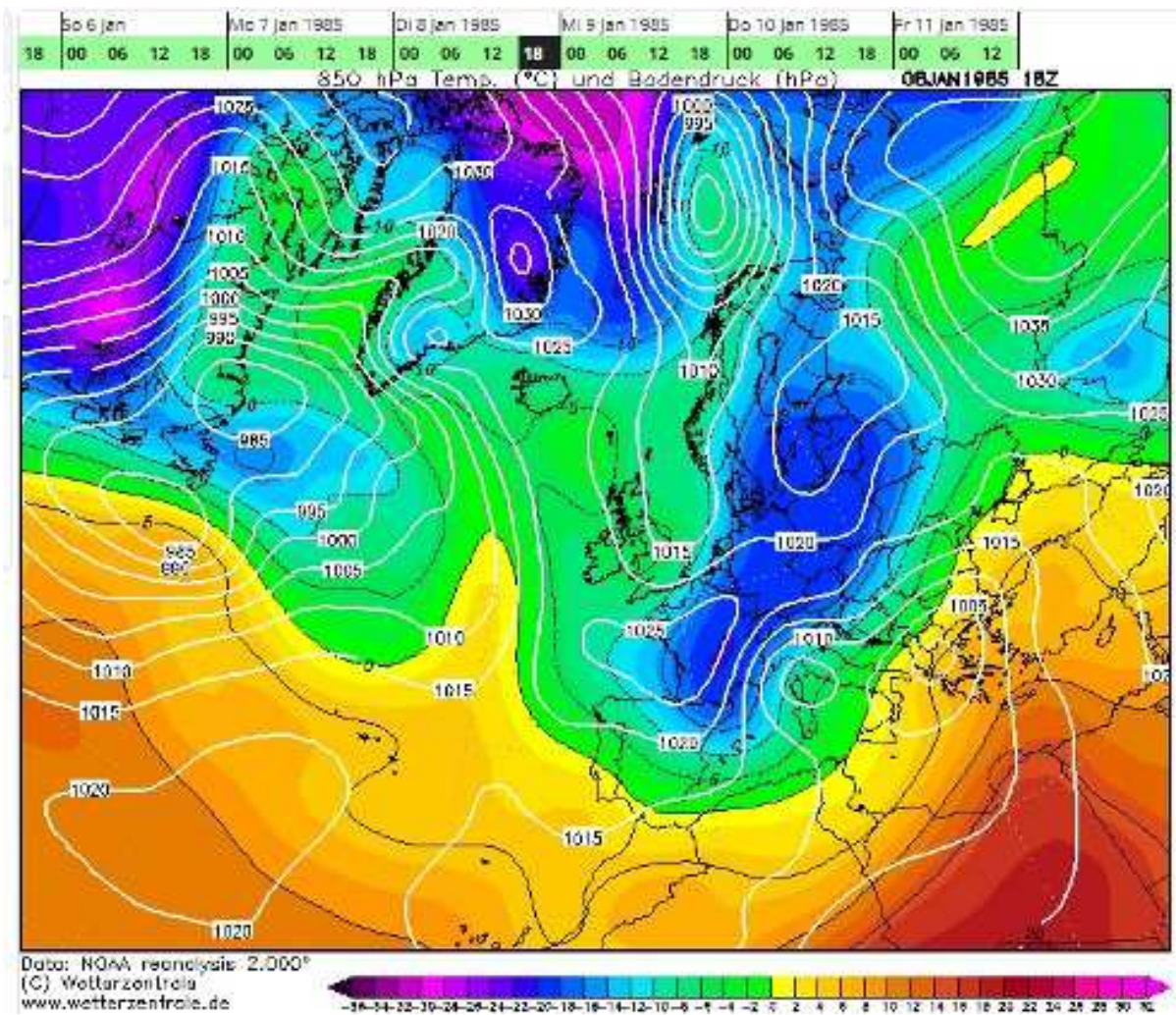
Mapa de superfície i 850 hPa del 8 de gener de 1985, a 18h.U.T.C. Es pot veure com la isoterma de -15^{\circ}\text{C} a 850 hPa la tenim a sobre. Font: wetterzentrale.de
