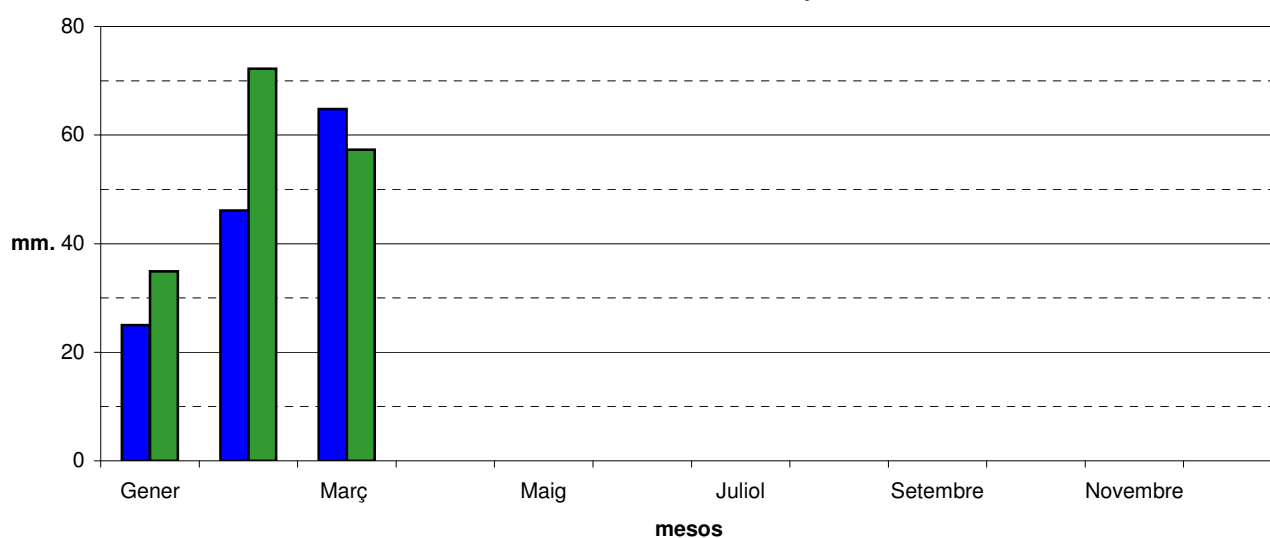
Pluviometria a l'Estartit i Torroella, any 2018
