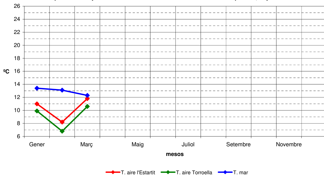
Temperatures mitjanes de l'aire a l'Estartit i Torroella i del mar en superfície, any 2018
