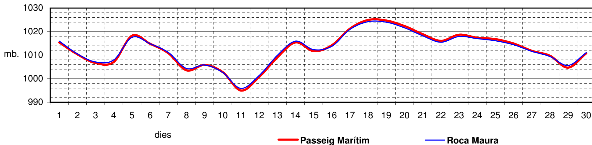
L'Estartit - Pressió atmosfèrica reduïda al nivell del mar - abril 2018
