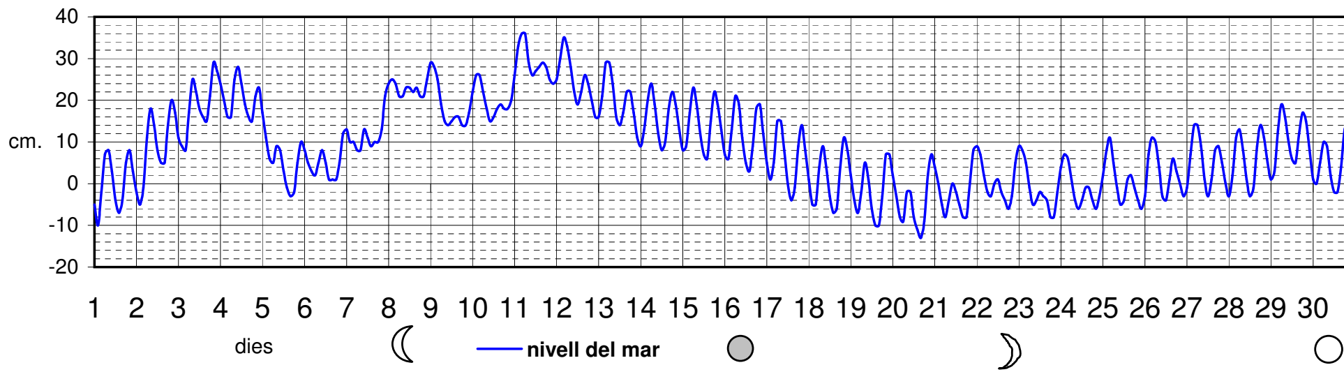
L'Estartit - marea - abril 2018
