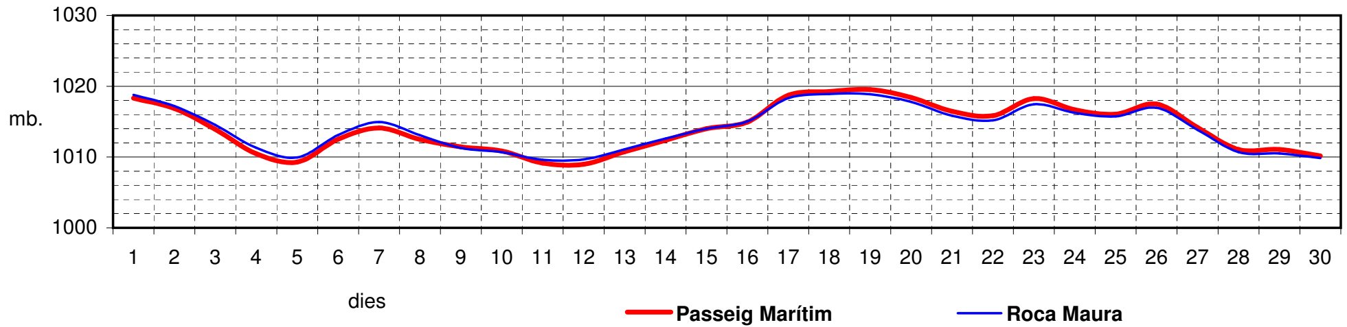
L'Estartit - Pressió atmosfèrica reduïda al nivell del mar - juny 2018
