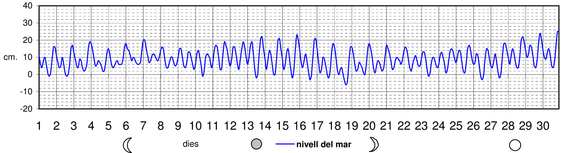
L'Estartit - marea - juny 2018
