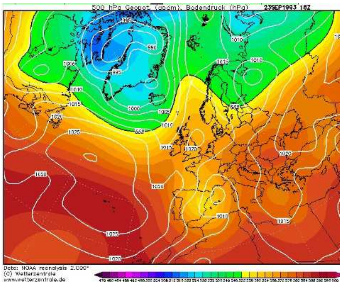
Mapa isobàric de les 18 UTC del 23 de setembre de 1993. Font: Wetterzentrale
