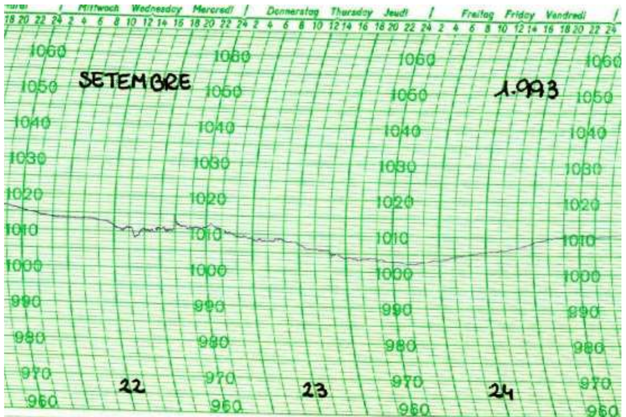
Barograma entre els dies 22 i 24 de setembre de 1993. Es pot observar una pressió atmosfèrica força baixa per aquelles dates.
