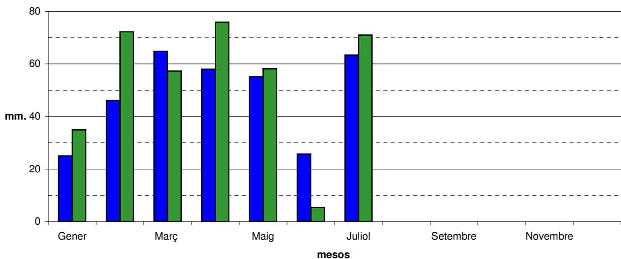
Pluviometria a l'Estartit i Torroella, any 2018
