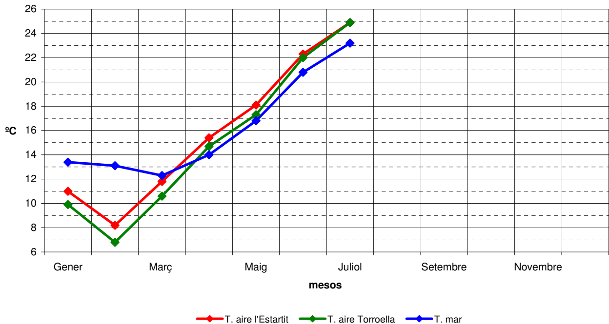
Temperatures mitjanes de l'aire a l'Estartit i Torroella i del mar en superfície, any 2018
