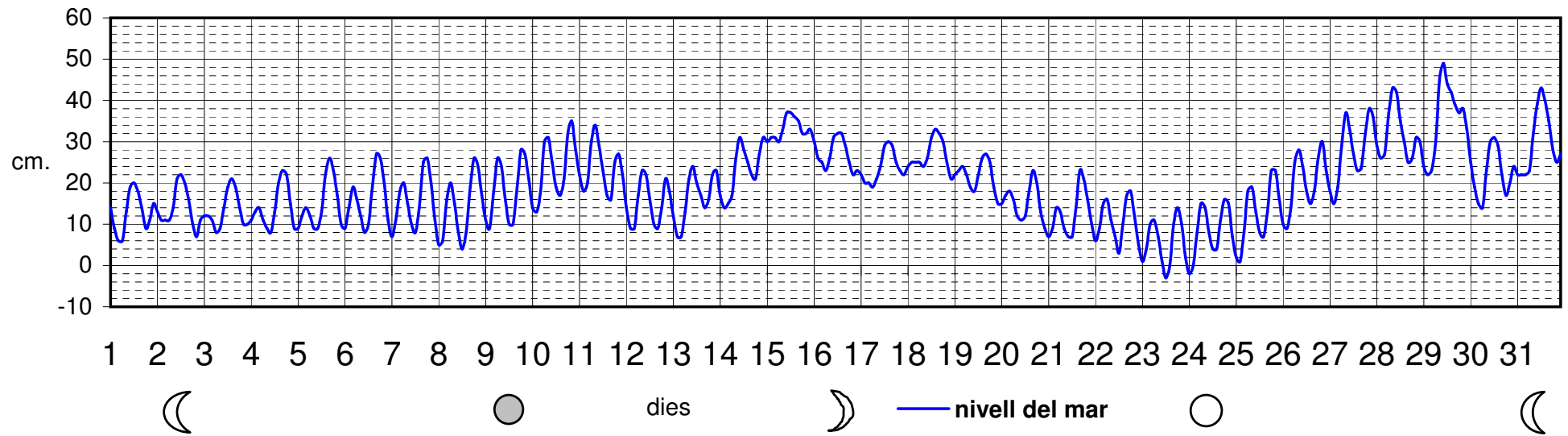
L'Estartit - marea - octubre 2018
