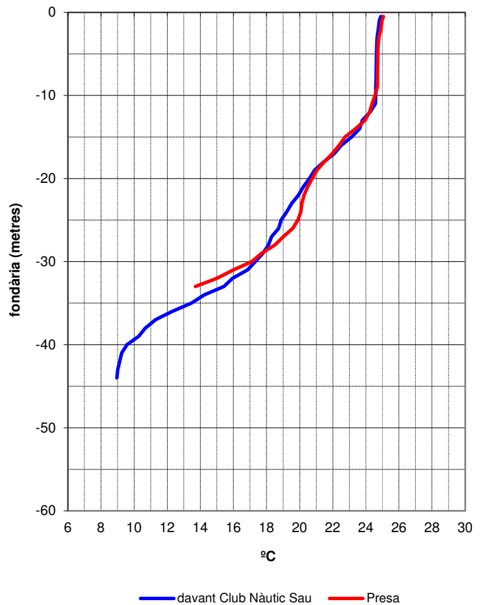
Temperatura de l'aigua del pantà de Sau - Dia 1 de setembre de 2021
