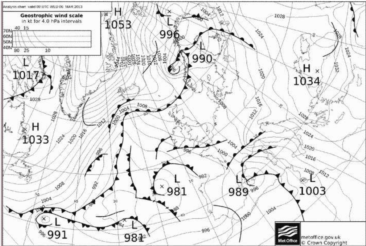
Mapa isobàric del 6 de març de 2013 a 00 UTC (font: Metoffice)
