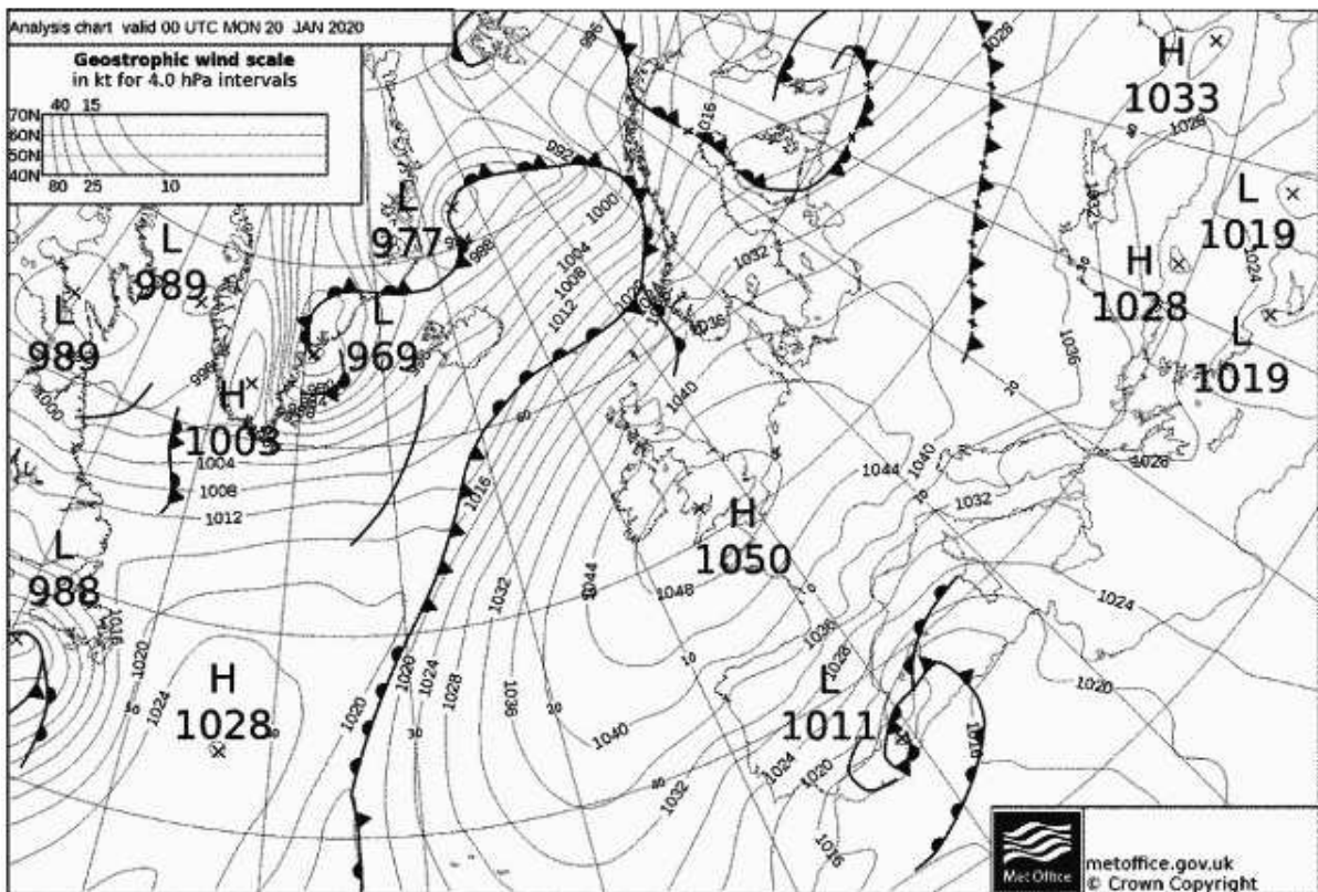
Situació isobàrica del 20 de gener de 2020. Es pot veure el fort gradient de pressió a la costa oriental peninsular. Font: Metoffice-Wetterzentrale.
