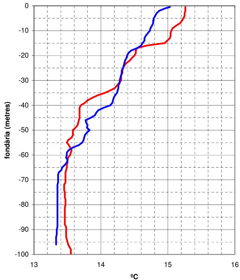
Temperatura del mar - Palamós 4 - l'Estartit 5 de maig de 2021
