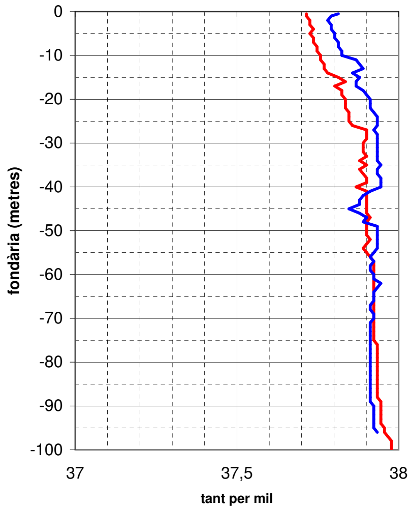
Salinitat del mar - Palamós 4 - l'Estartit 5 de maig de 2021
