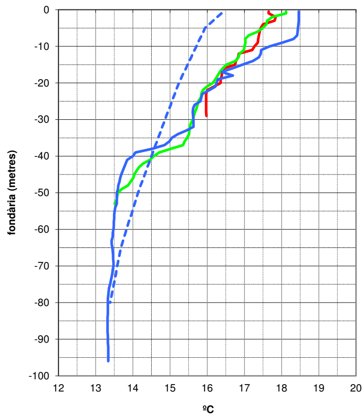
Temperatura del mar - Zona de les Medes - Dia 20 de maig de 2022
