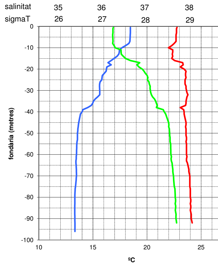
Temperatura i salinitat del mar - Una milla a llevant de les Medes - 20 de maig de 2022
