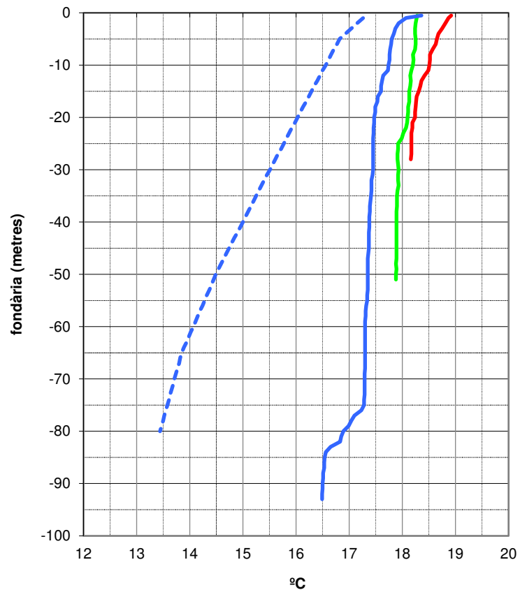
Temperatura del mar - Zona de les Medes - Dia 28 de maig de 2022
