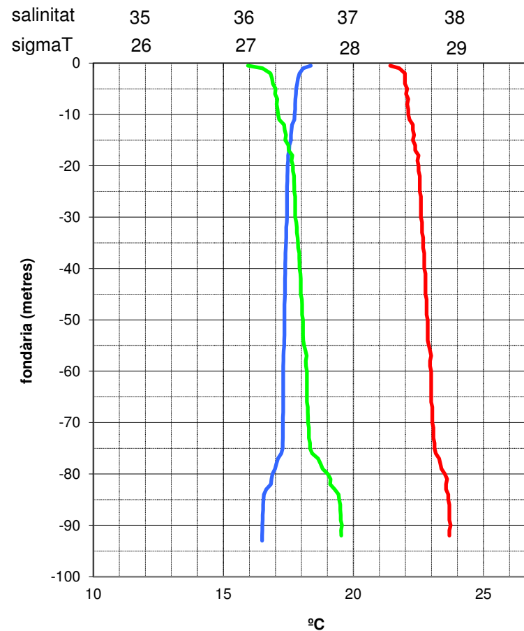
Temperatura i salinitat del mar - Una milla a llevant de les Medes - 28 de maig de 2022
