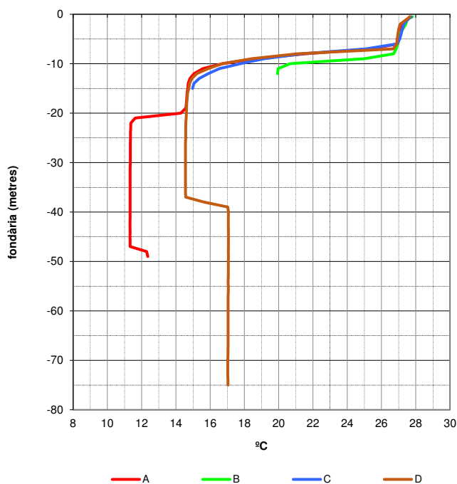
Temperatura de l'aigua de l'estany de Banyoles - Dia 11 de juliol de 2022
