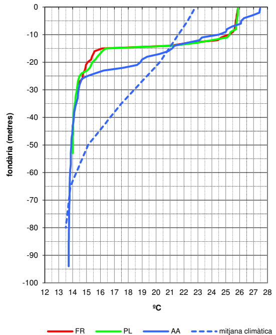
Temperatura del mar - Zona de les Medes - Dia 4 d'agost de 2022
