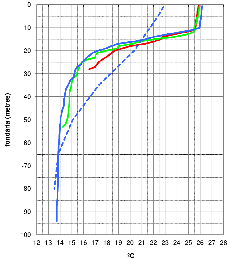
Temperatura del mar - Zona de les Medes - Dia 8 d'agost de 2022
