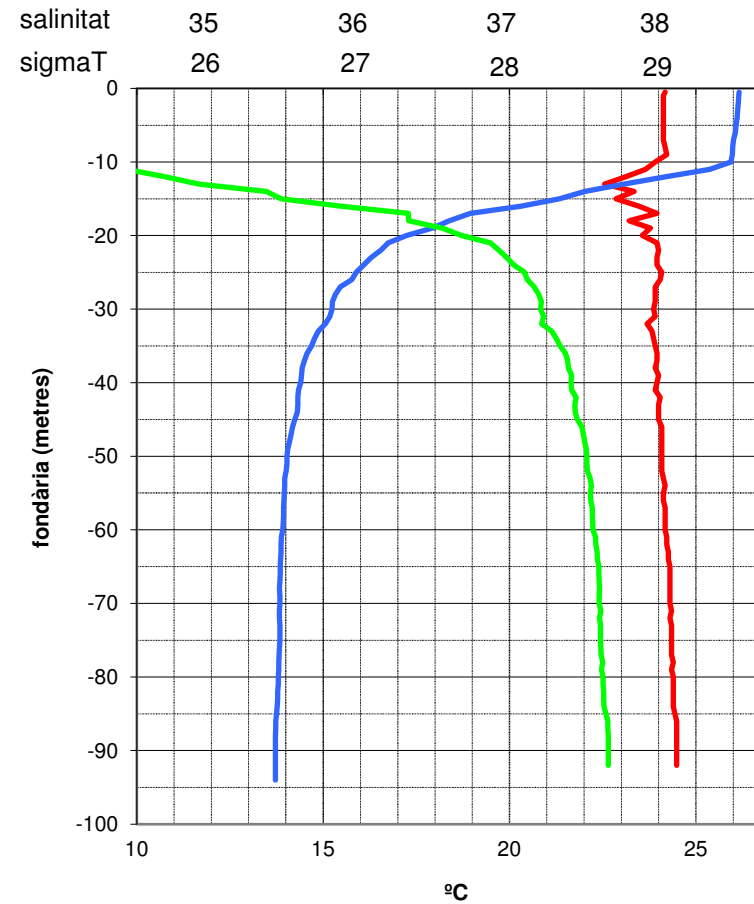
Temperatura i salinitat del mar - Una milla a llevant de les Medes - 8 d'agost de 2022
