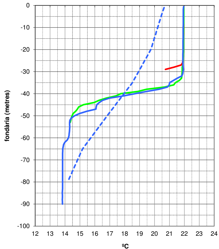
Temperatura del mar - Zona de les Medes - Dia 22 de setembre de 2022
