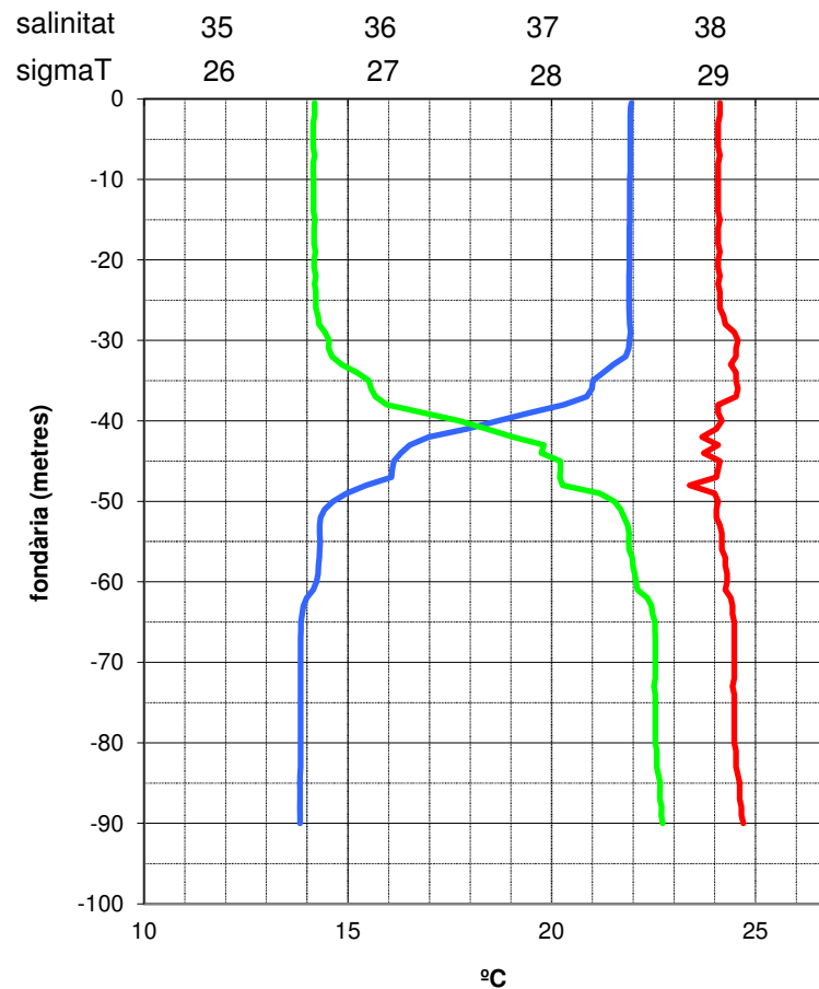
Temperatura i salinitat del mar - Una milla a llevant de les Medes - 22 de setembre de 2022
