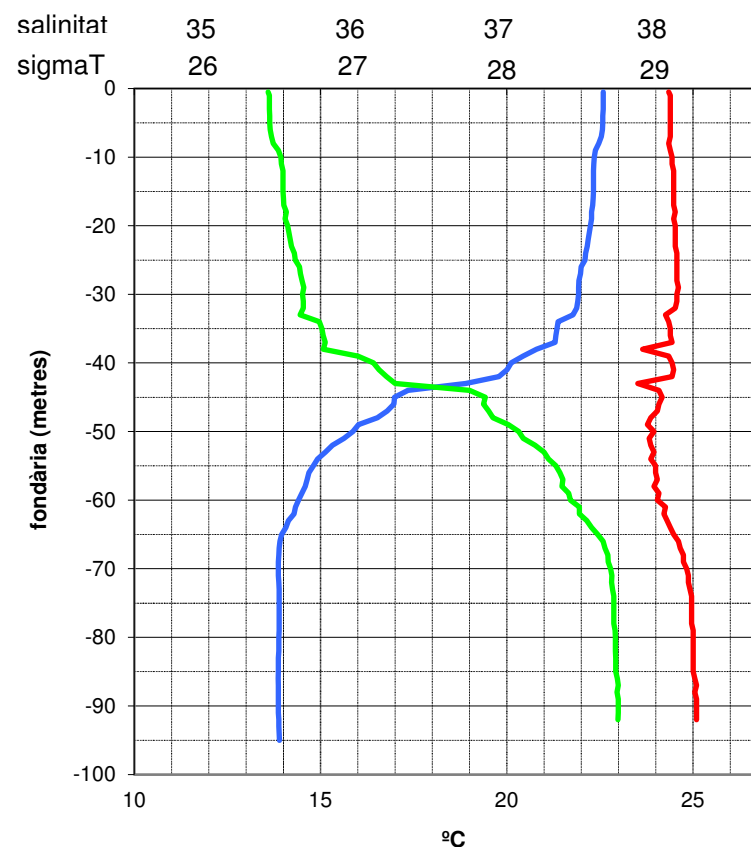
Temperatura i salinitat del mar - Una milla a llevant de les Medes - 1 d'octubre de 2022
