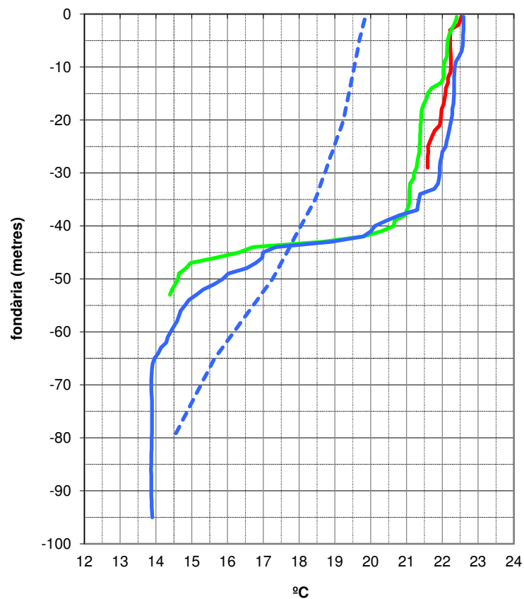
Temperatura del mar - Zona de les Medes - Dia 1 d'octubre de 2022
