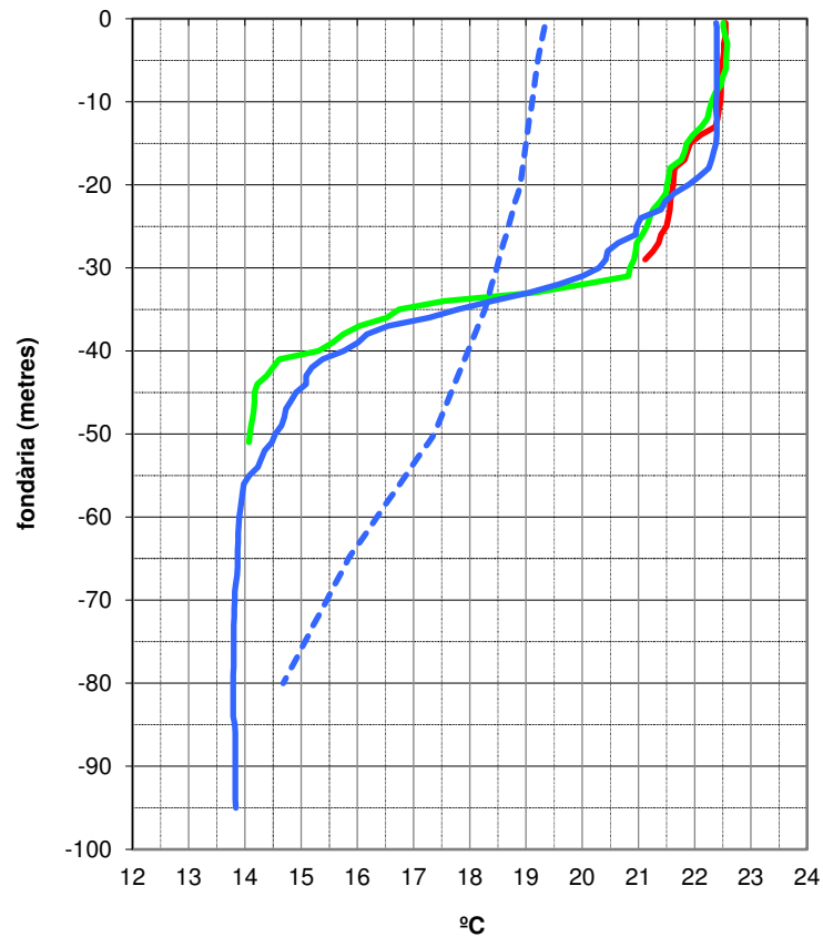
Temperatura del mar - Zona de les Medes - Dia 7 d'octubre de 2022
