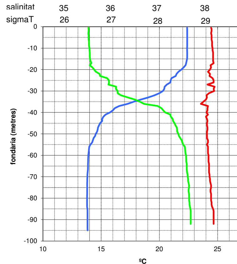
Temperatura i salinitat del mar - Una milla a llevant de les Medes - 7 d'octubre de 2022
