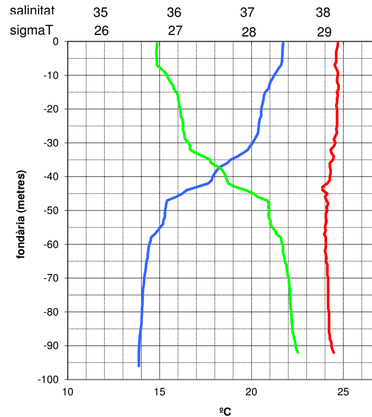
Temperatura i salinitat del mar - Una milla a llevant de les Medes - 14 d'octubre de 2022
