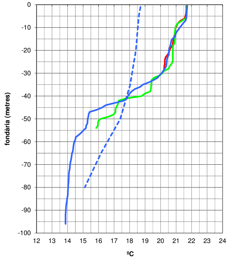
Temperatura del mar - Zona de les Medes - Dia 14 d'octubre de 2022
