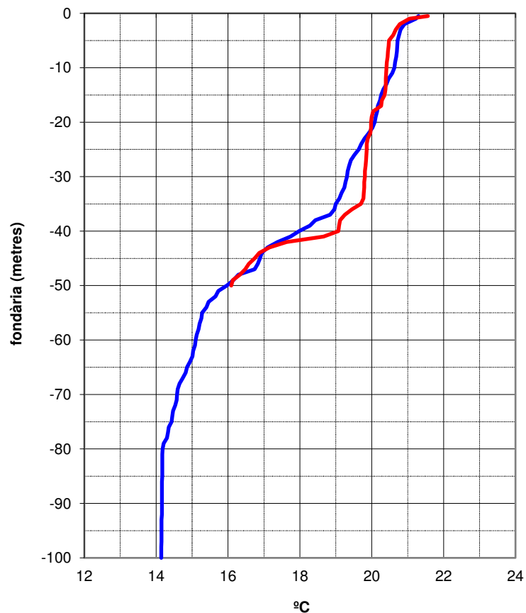
Temperatura del mar - Palamós - 18 d'octubre de 2022
