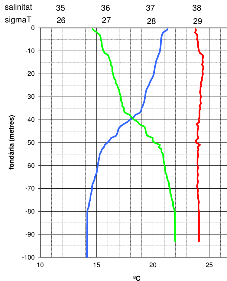
Temperatura i salinitat del mar - 18 d'octubre de 2022
